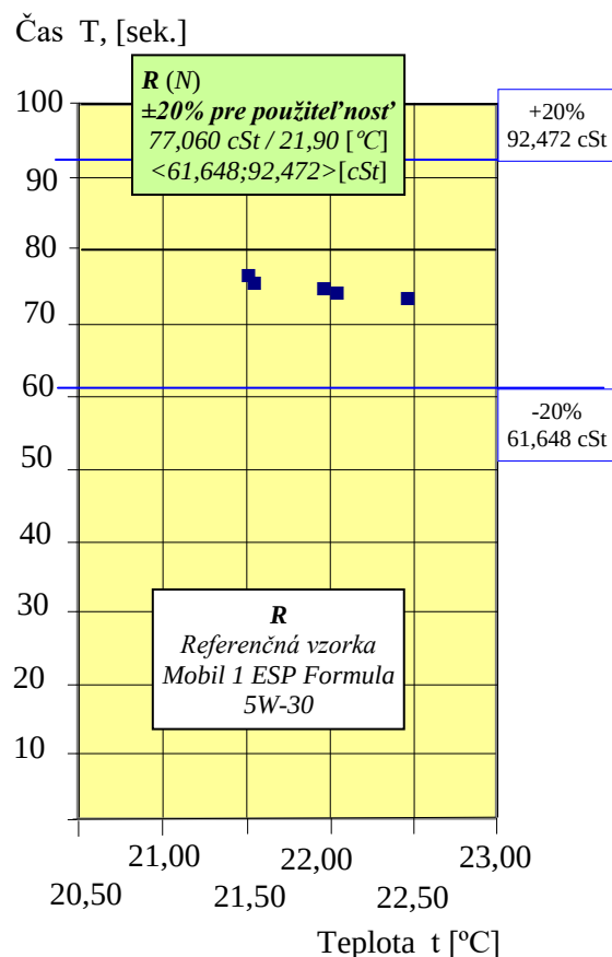
Diagram „ka“ hodnotenia kinematickej viskozity (priemer kalibračnej konštanty - prietokovej dýzy = 3 \text{ mm}^2 )
