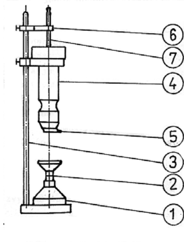
Obr.:Schéma viskozimetra
